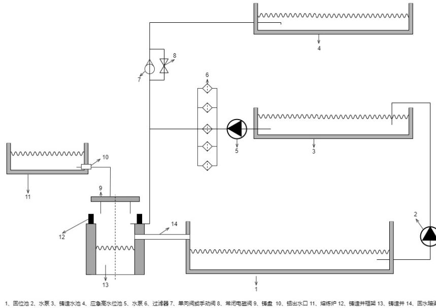
图A.1 半连续（深井）铸造冷却水循环系统（一般）示意图
