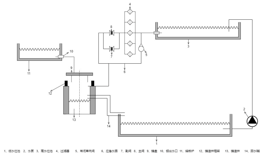
图A.2 半连续（深井）铸造冷却水循环系统（铸造冷却水池为高位水池）示意图
